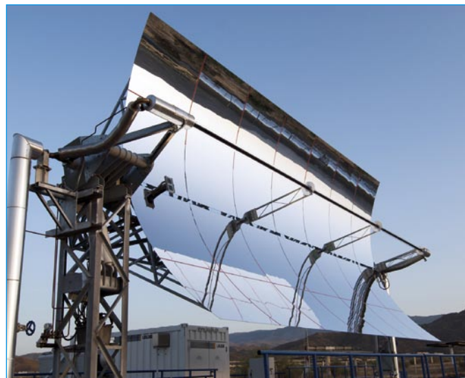
Proyecto KONTAS, en la Plataforma Solar de Almería. KONTAS project at the Plataforma Solar de Almería.
